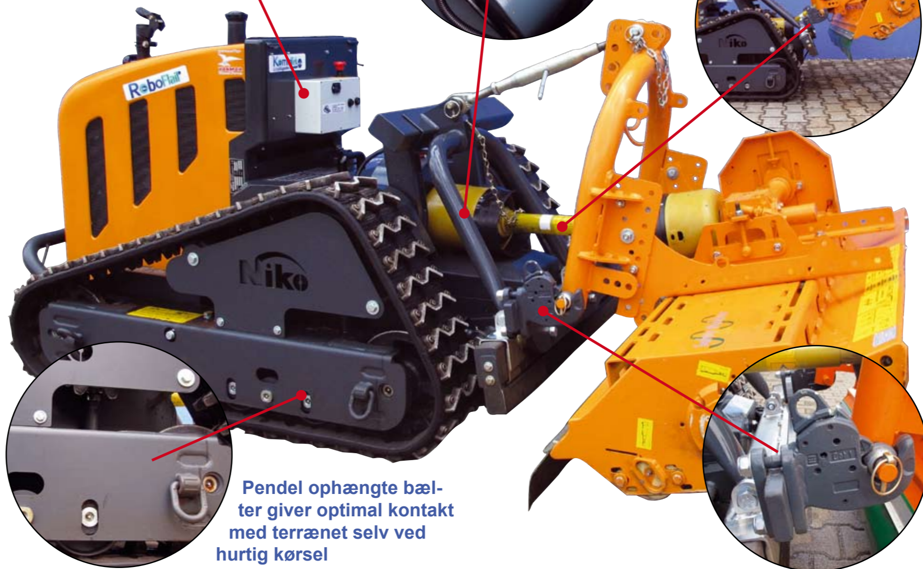
Redskabsophæng kategori 1 - standardsystem til påmontering af dine liftofhængte redskaber
