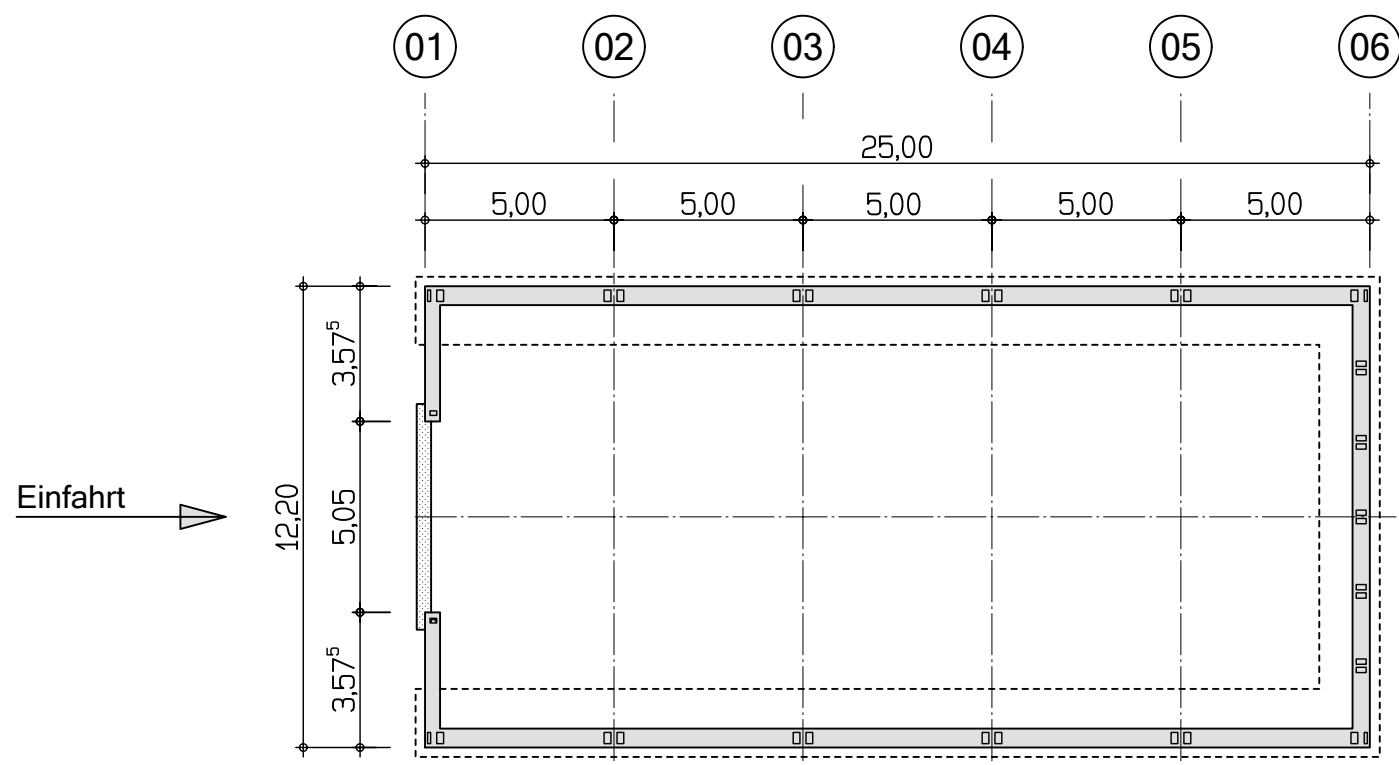
Grundriss Hallenfundament
